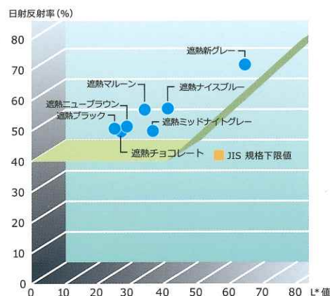
図2. 近赤外波長域日射反射率
